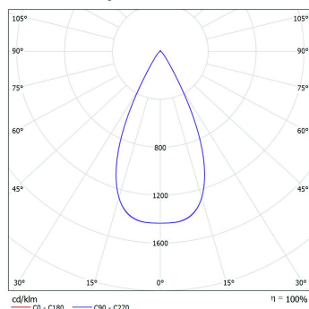
Abstrahlwinkel 50°
