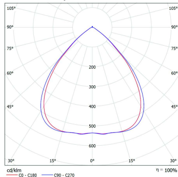
Abstrahlwinkel 90°
