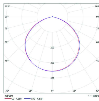
Abstrahlwinkel 120°
